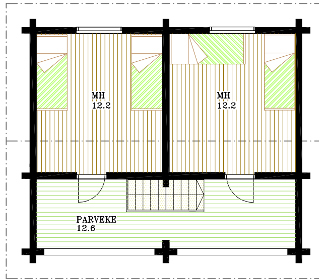
POHJAPIIRROS II-KERROS
