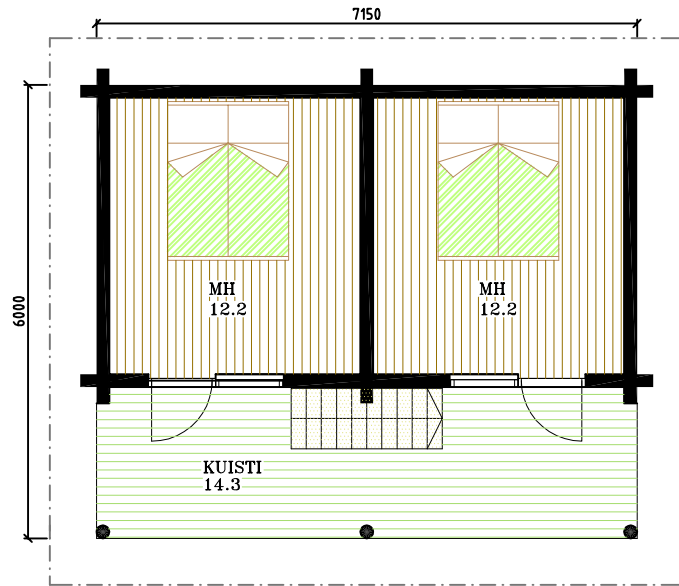
POHJAPIIRROS I-KERROS
